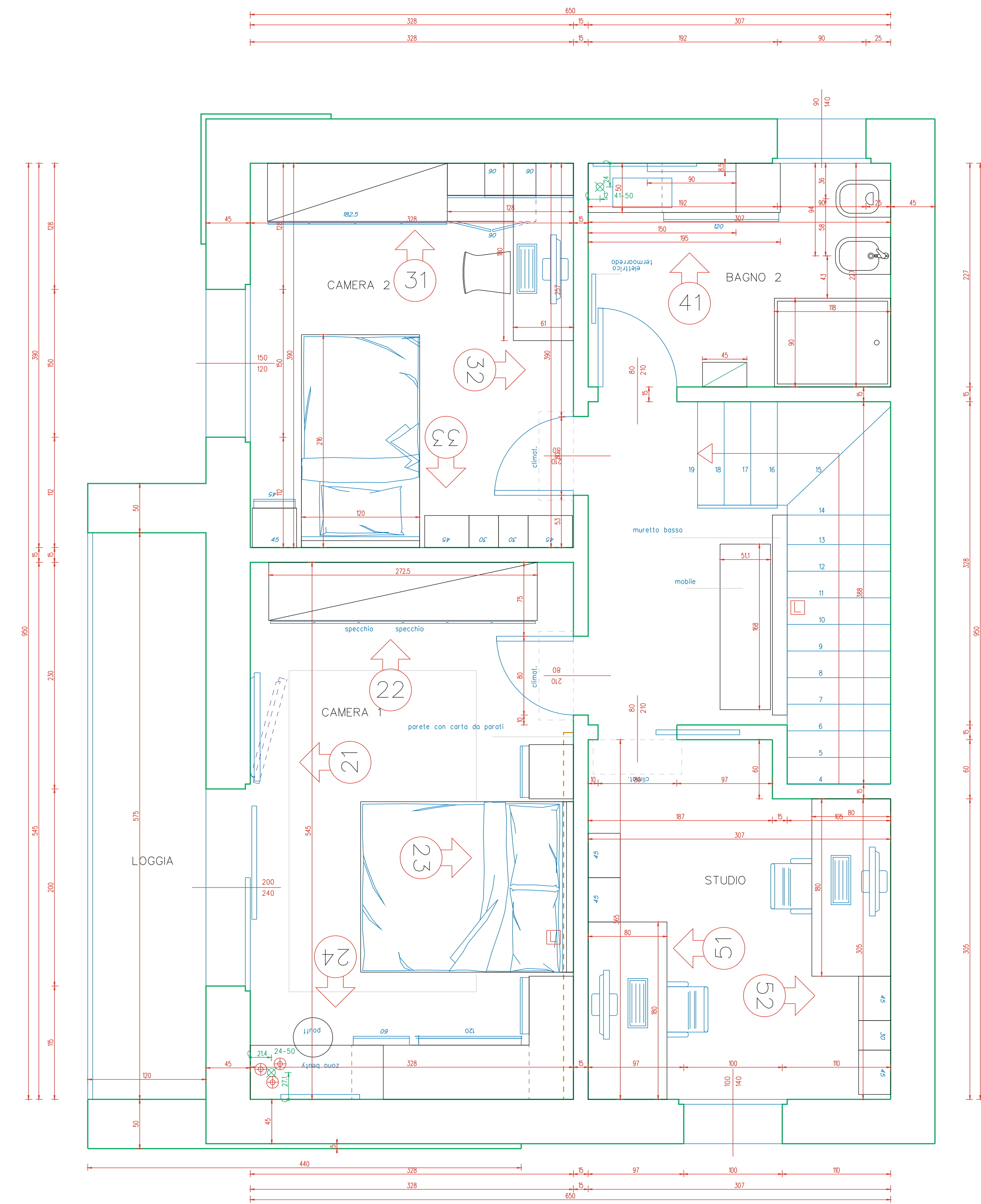
PRIMO PIANO - V 5.0 (da costruttore)
