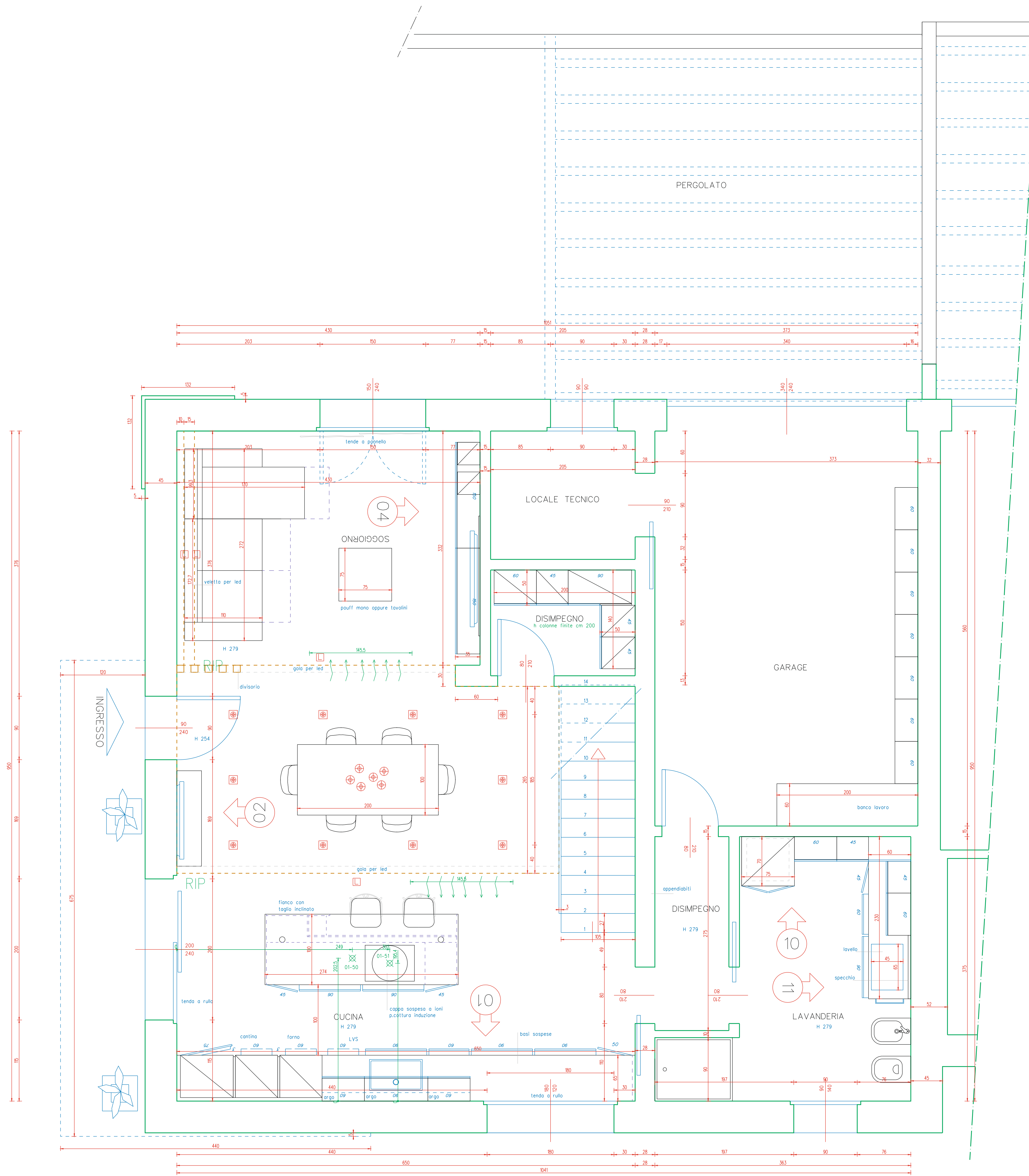
PIANO TERRA - V 5.0 (da costruttore)
