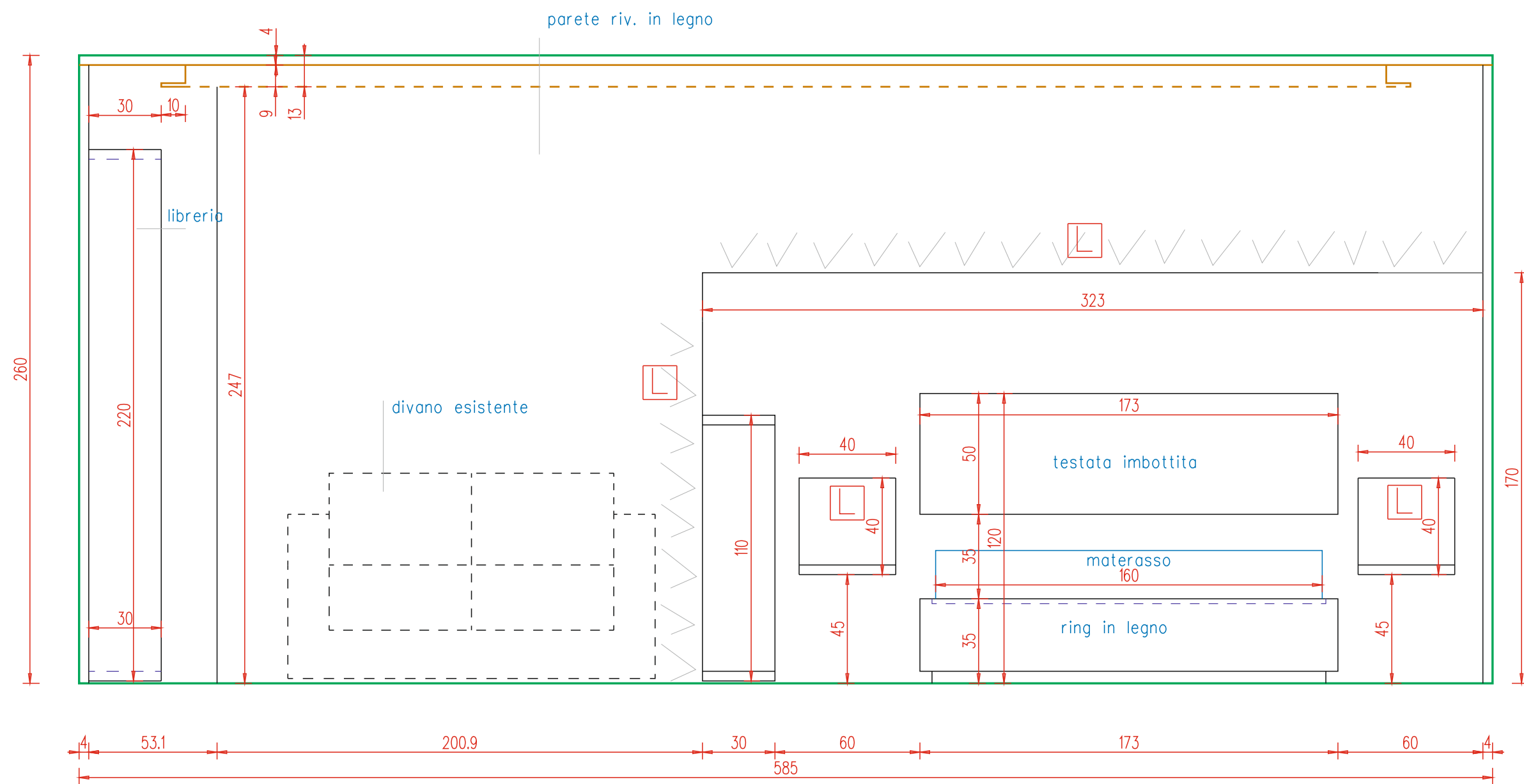
PROSPETTO - A
