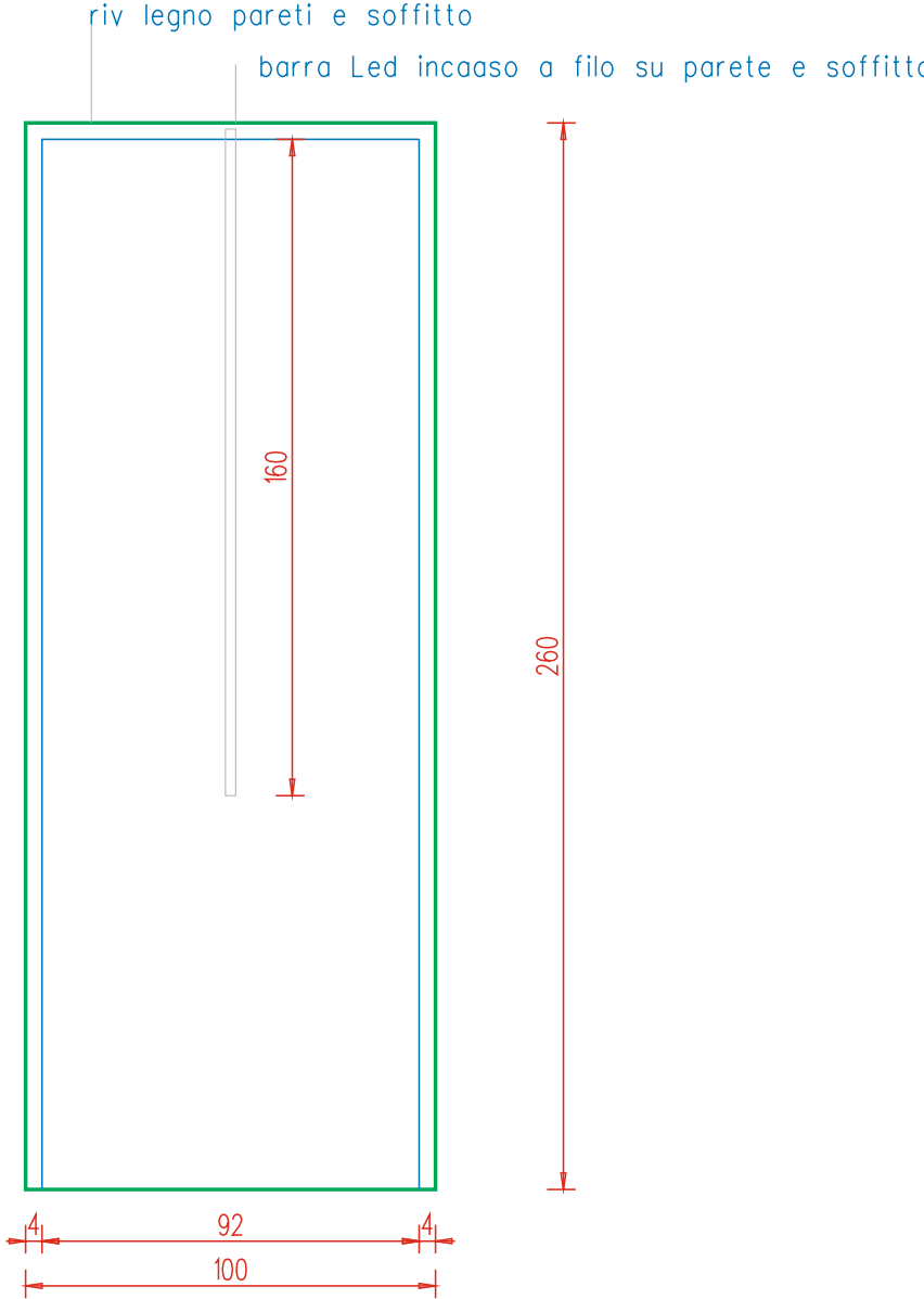
PROSPETTO - E
