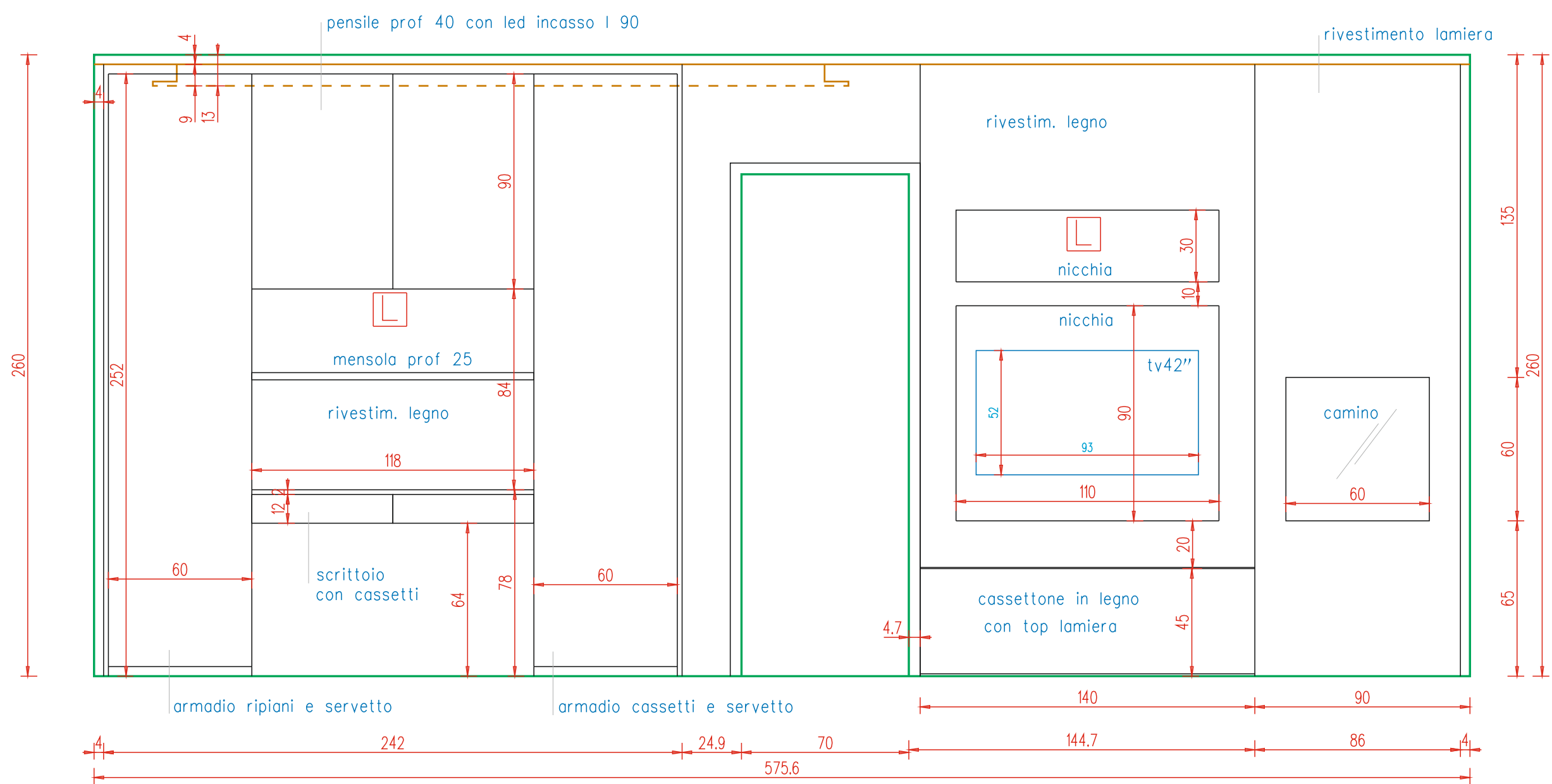
PROSPETTO - B
