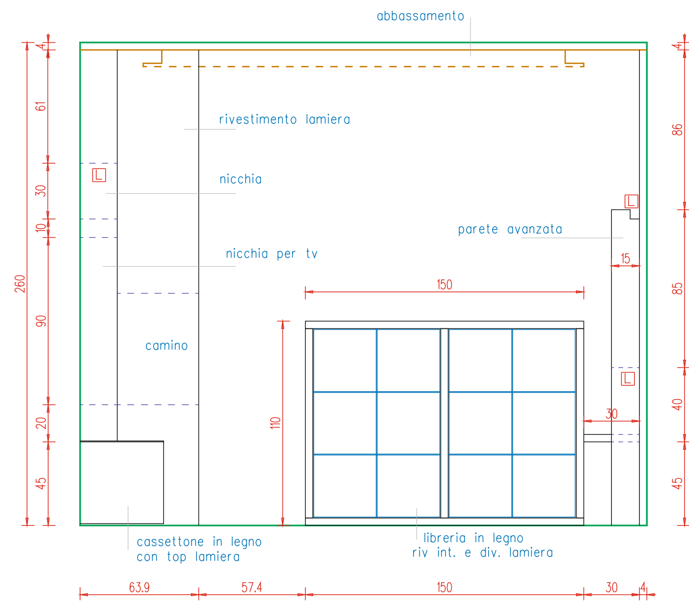
PROSPETTO - C
