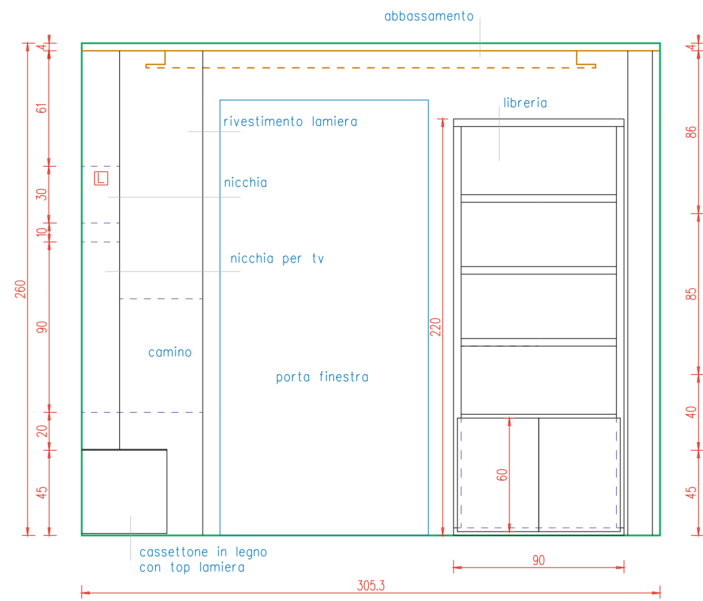
PROSPETTO - D
